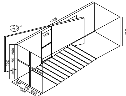
図 1-2 光の教会のアイソメ図
